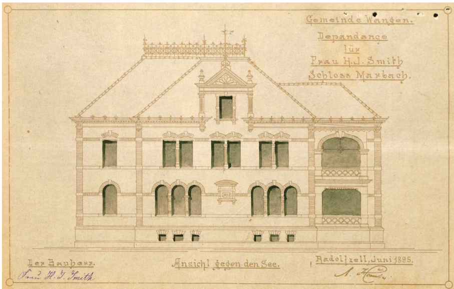
Aufriss der Villa Bella Vista aus dem Baugesuch von 1895 (Staatsarchiv Freiburg B 715/1 Nr. 965, Baugesuche, Nr. 54)
