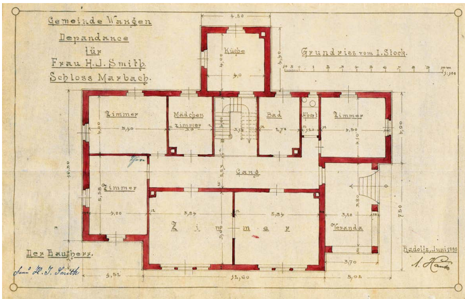
Grundriss der Villa Bella Vista (Staatsarchiv Freiburg B 715/1 Nr. 965, Baugesuche, Nr. 57)
