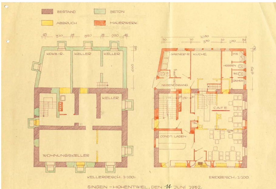
Grundriss des Erdgeschosses mit Ladenausstattung nach den Umbauplänen im Jahr 1932 (Zentralregistratur der Stadt Singen, Bauakte)
